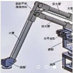
码垛机械手
